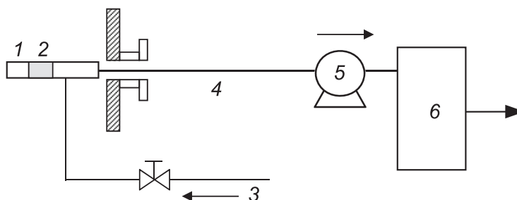
Рисунок В.1 — Схема горячей оптической измерительной системы (пример)
